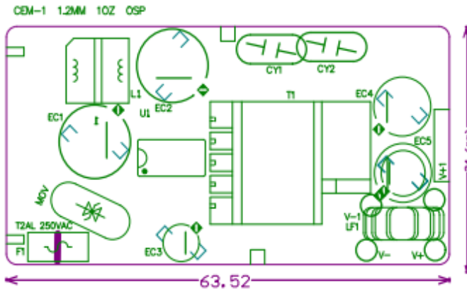
TOP OVERLAY
