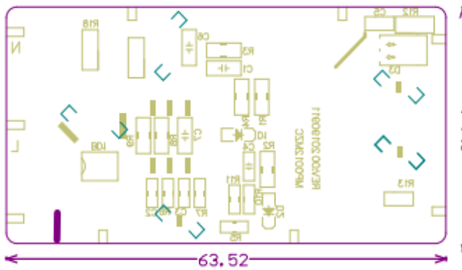
BOTTOM OVERLAY
