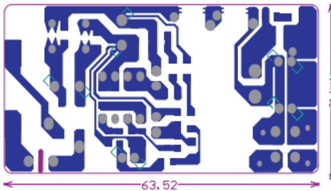
BOTTOM LAYER
